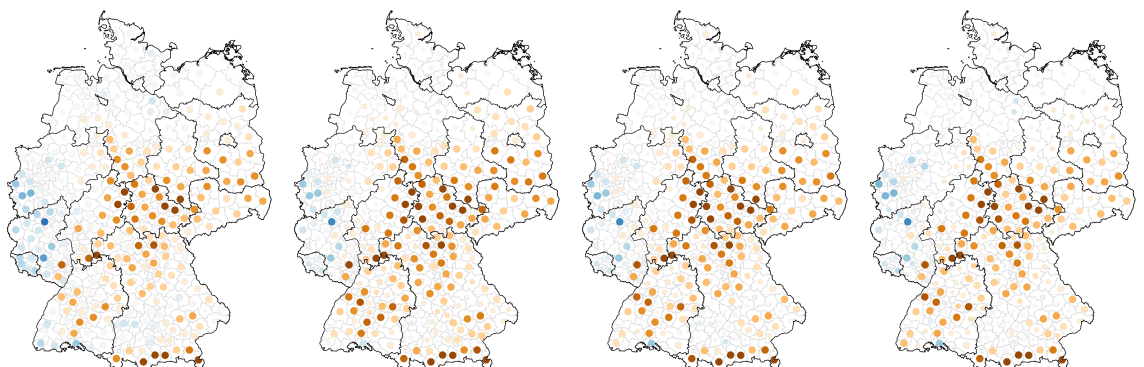
Abb. 3: Saisonale Vorhersagen (2025-Dez bis 2026-Jun) ; Mittel der Anomalien des gesamten Bodenwasserspeichers, ParFlow/CLM Simulationen (initialisiert: 2025-12-01) mit ECMWF SEAS Antrieb (50 Ensemble Member). Punkte: NUTS-3 Verwaltungsebene; Punktgröße: Proportional der Anzahl der Member mit identischem Vorzeichen (positive oder negative Anomalie).
